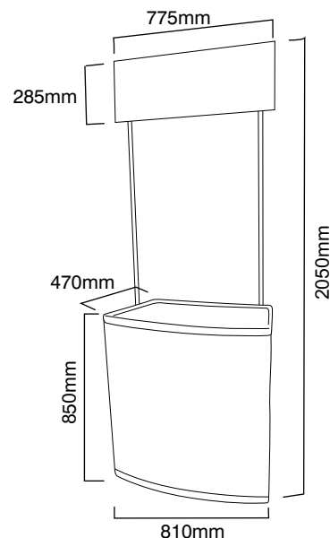
Rozměry sestaveného stolku
